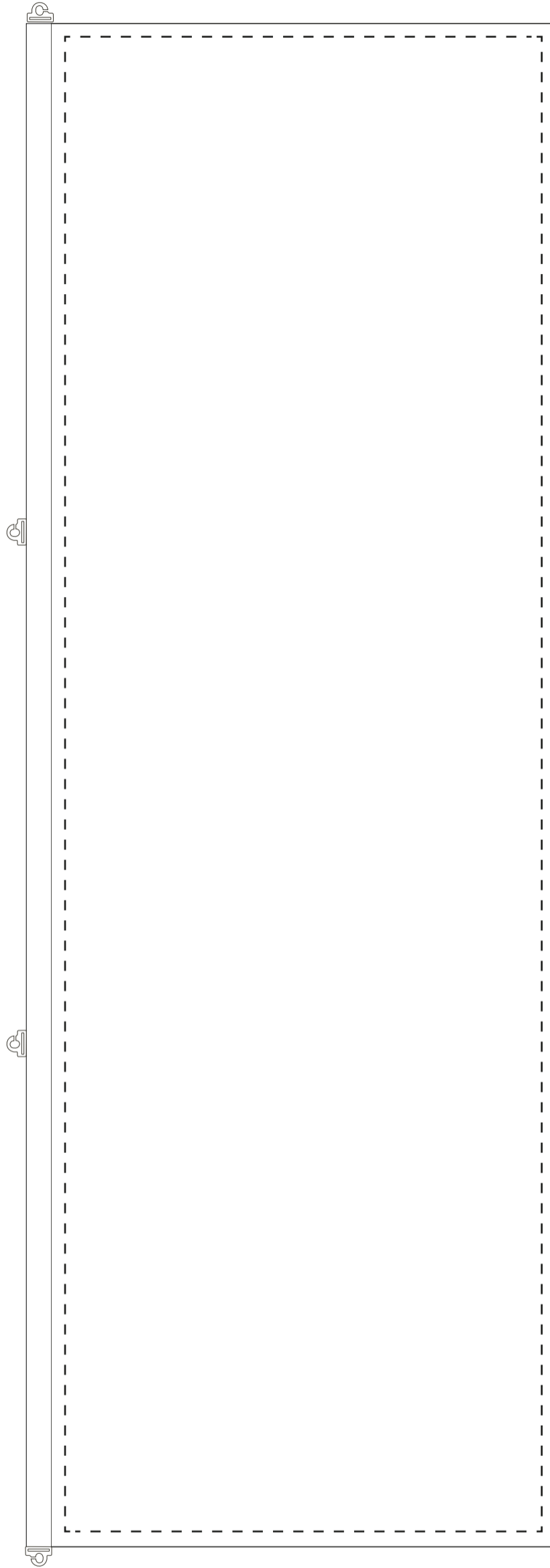
Flagga 100 x 300 cm 30 mm sömsmån, Skala 1:10
